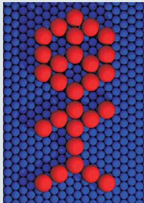
Diese Illustration zeigt den wohl kleinsten Zwerg der Welt, der von dem amerikanischen Physiker Don Eigler bei IBM mit Hilfe eines Rastertunnelmikroskops aus 28 Kohlenmonoxid-Molekülen auf einer Platinoberfläche erzeugt wurde.
