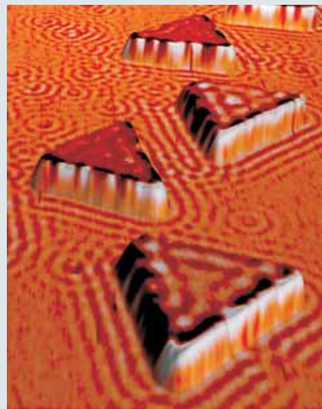
Kobaltinseln mit einer Höhe von zwei atomaren Lagen auf einer Kupferoberfläche. Die wellenartigen Muster sind Interferenzen der Elektronenwellen, welche an den Kobaltinseln und anderen Defekten im Kristall gestreut werden. Die Aufnahme wurde mit einem Rastertunnelmikroskop gemacht.
