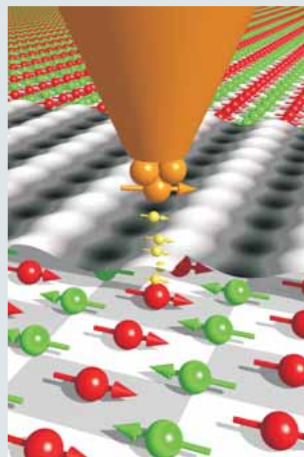
Eine schematische Abbildung, die das Experiment beschreibt, in dem mit dem Spinpolarisierten Rastertunnelmikroskop die magnetischen Eigenschaften einzelner Atome sichtbar gemacht wurden.
