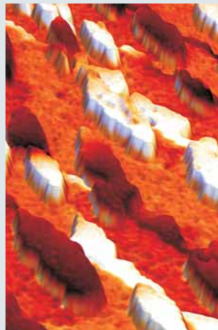
„Canyonlandschaften“ aus atomaren „Eisenbergen“, die gerade mal ein Atom hoch und zum Teil nur 10 bis 20 Atome breit sind. Helle Flächen entsprechen dem magnetischen Nord-, die dunklen dem magnetischen Südpol.
