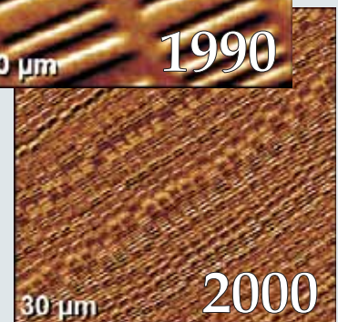
Die Abbildung zeigt die Entwicklung der Abmessungen von Bit-Strukturen in den letzten zwanzig Jahren (© IBM).
